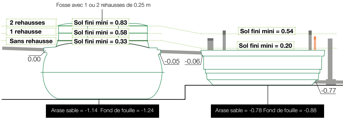
Profil type des versions 5 et 7 EH
