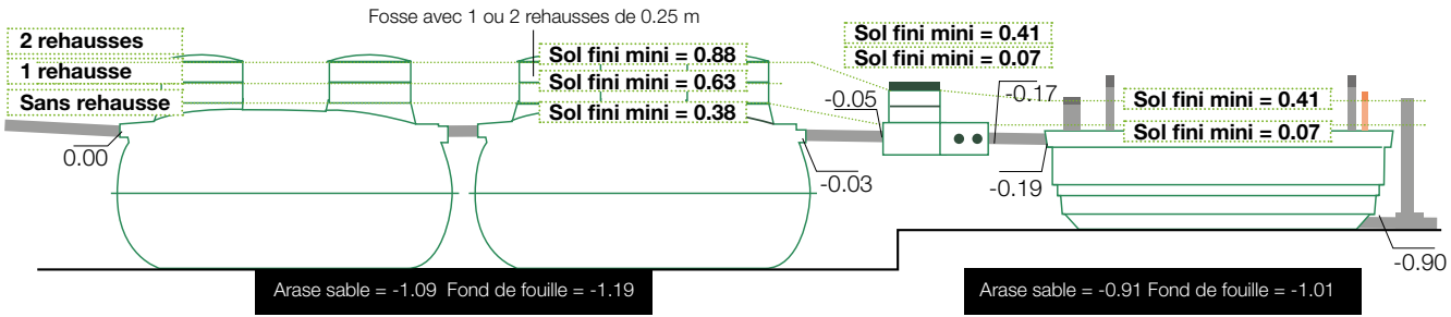
Profil type des versions 8/15 et 16/20 EH
