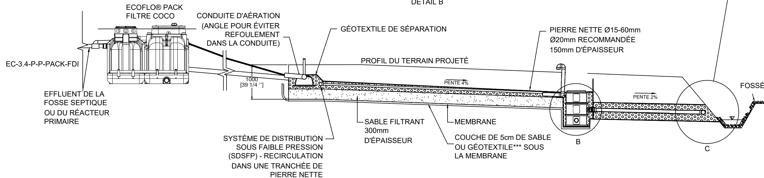
COUPE A-A
