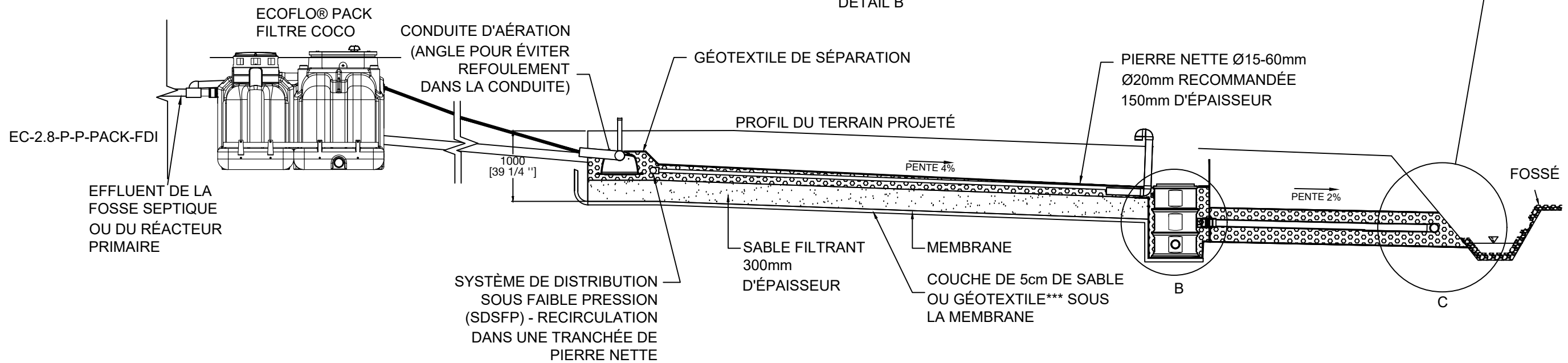
COUPE A-A
