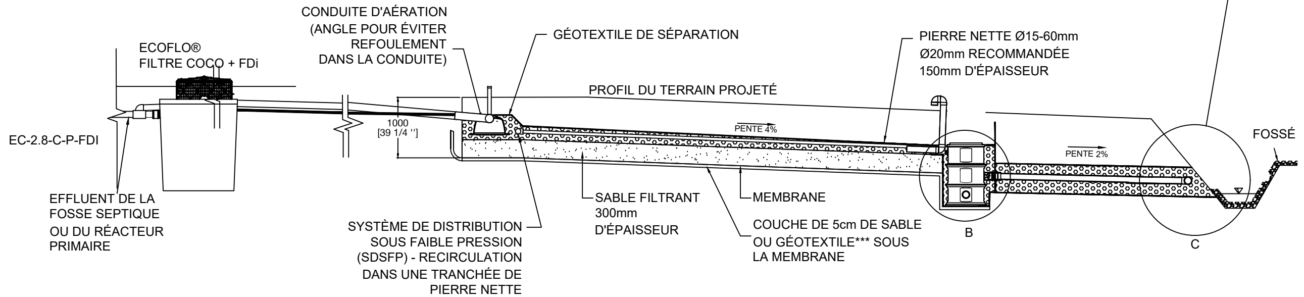
COUPE A-A
