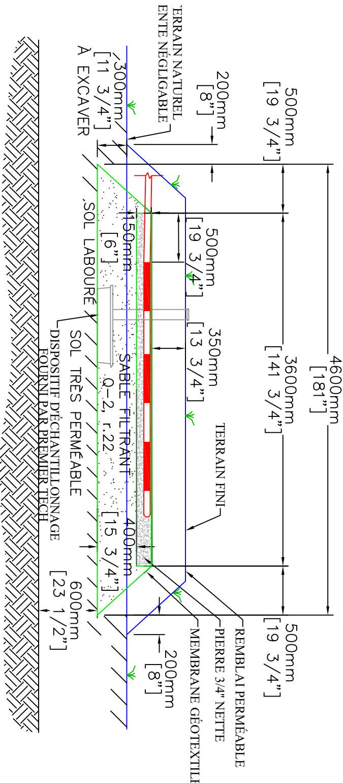
COUPE LONGITUDINALE
