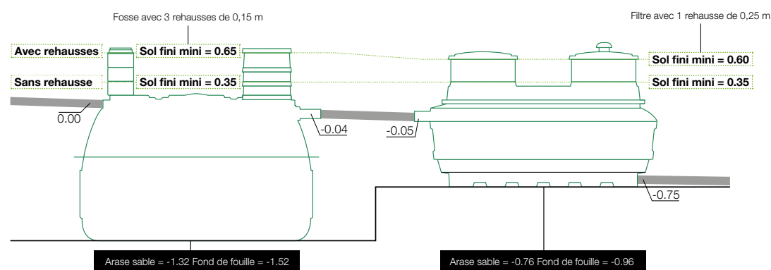
Filière 6 EH / Fosse de 4 m 3 + filtre de 6 m 2
