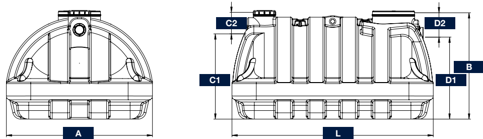
Fosse 3, 4 et 5 m³ - EPARCO filière plate écorces de pin 4 à 10 EH
