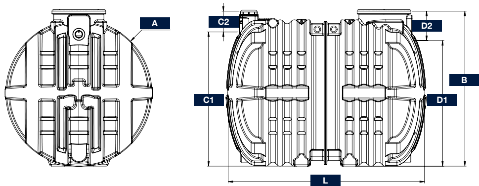
Fosse 6 m³ - EPARCO filière plate écorces de pin 12 EH
