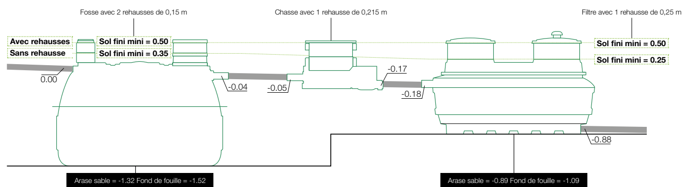
Filière 7 EH / Fosse de 4 m 3 + 2 filtres de 4 m 2
