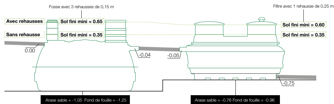
Filière 4 et 5 EH / Fosse de 3 m 3 + filtre de 4 ou 5 m 2
