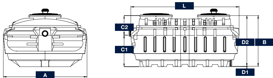
Filtres 4, 5 et 6 m²
